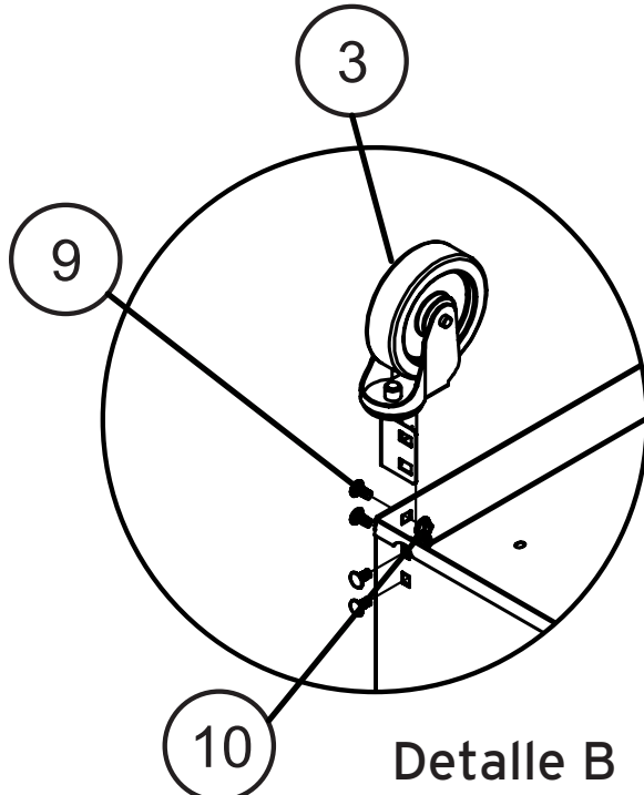
Detalle B
